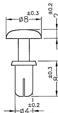
SNAP RIVET SCALE 2:1
