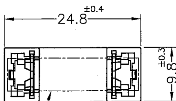
FOR FUSE(φ5X20)
