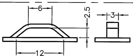
MONTAGEBOHRUNG 裝配件(尺寸僅供參考)
