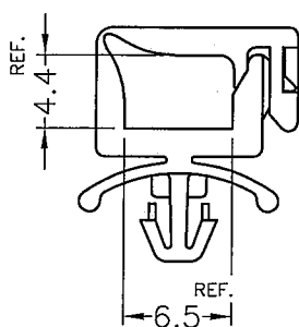
CLOSE DIAGRAM 扣合示意圖
