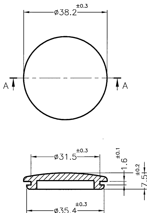
SECTION A-A
