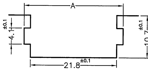
EDGE INSTALLATION
