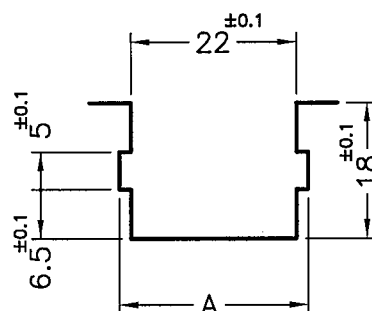
EDGE INSTALLATION
