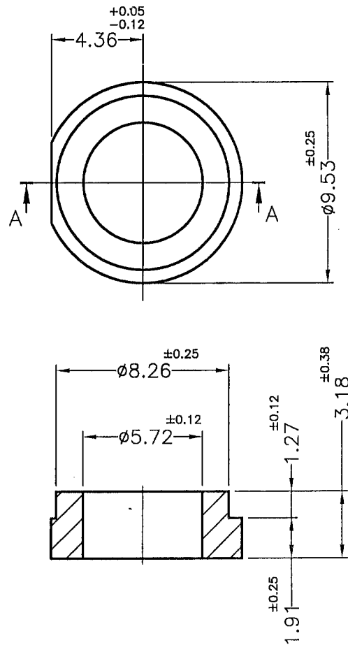
SECTION A-A
