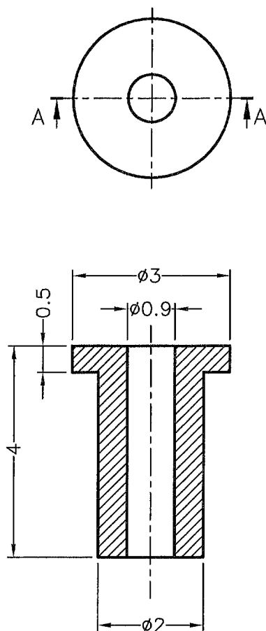
SECTION A-A
