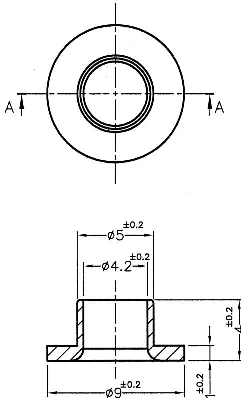
SECTION A-A
