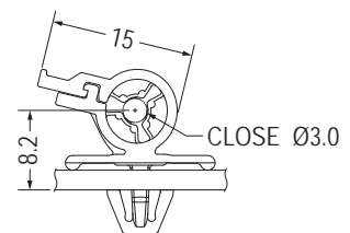
裝配示意圖 Assembly Diagram
