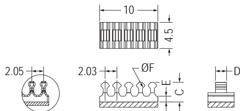
【MU-03L-4】 3M DOUBLE ADHESIVE TAPE
