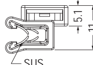
裝配示意圖 Assembly Diagram
