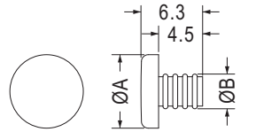
MOUNTING HOLE: ØG or M4 【 MHD-3.3 】
