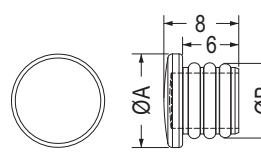
MOUNTING HOLE: ØG • Material: Silicon Rubber 【 MHD-7.5I 】
