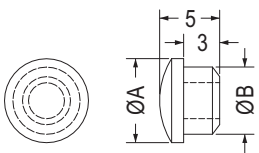
MOUNTING HOLE: ØG 【 MHD-5.5, MHD-5.5I 】
