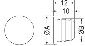
MOUNTING HOLE: ØG • Material: Silicon Rubber 【 MHD-17I 】
