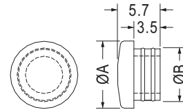
MOUNTING HOLE: ØG
