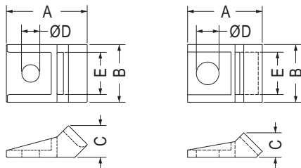
【 MTAB-4, MTAB-6 】 Mounting Screw Size
